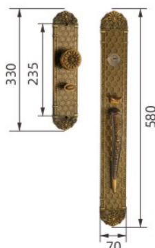
9802L-01单拉 黄古铜 Yellow Brass
