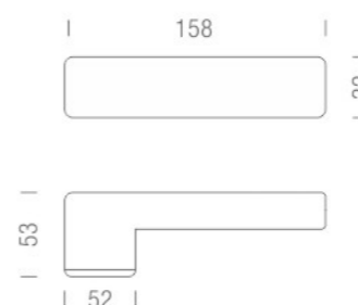
K20 OW Material: Zinc alloy
