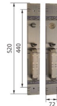
9806XL-05双拉 亚光青古铜 Matte Bronze
